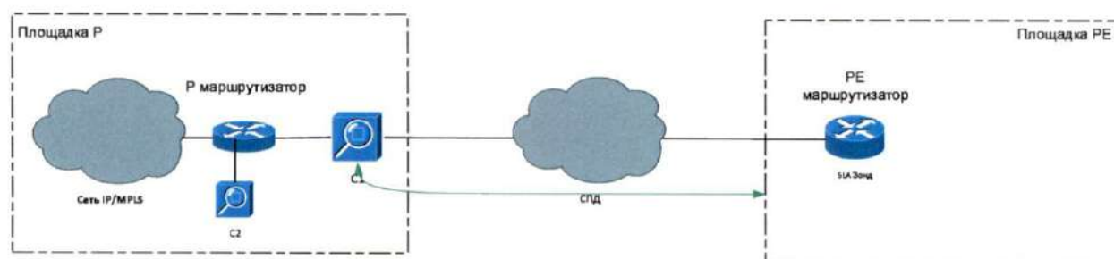
Рис.3. Типовые схемы подключения зондов на площадке типа Р
